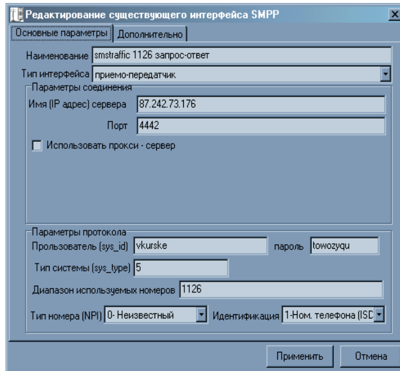
Диалог редактирования шлюза
