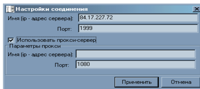
Окно настроек подключения
