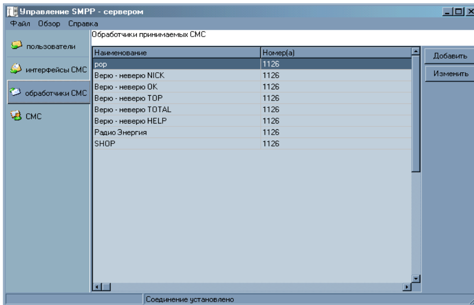
Вкладка «Обработчики СМС»
